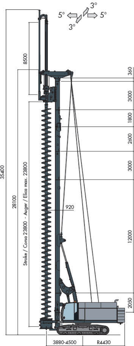
EXTENDED VERSION VERSIONE LUNGA
