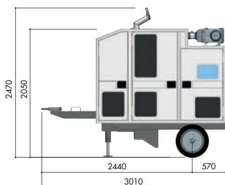
Power pack with diesel engine Centrale idraulica con motore diesel ~2100 kg
